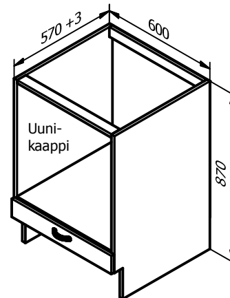
A6U ES 95 Huom! Vain metabox-laatikolla
