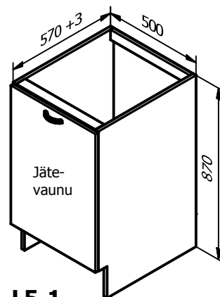
L5-1 Ovi 703 Kost. kestävä Laat. syv. 450 1 irtohylly
